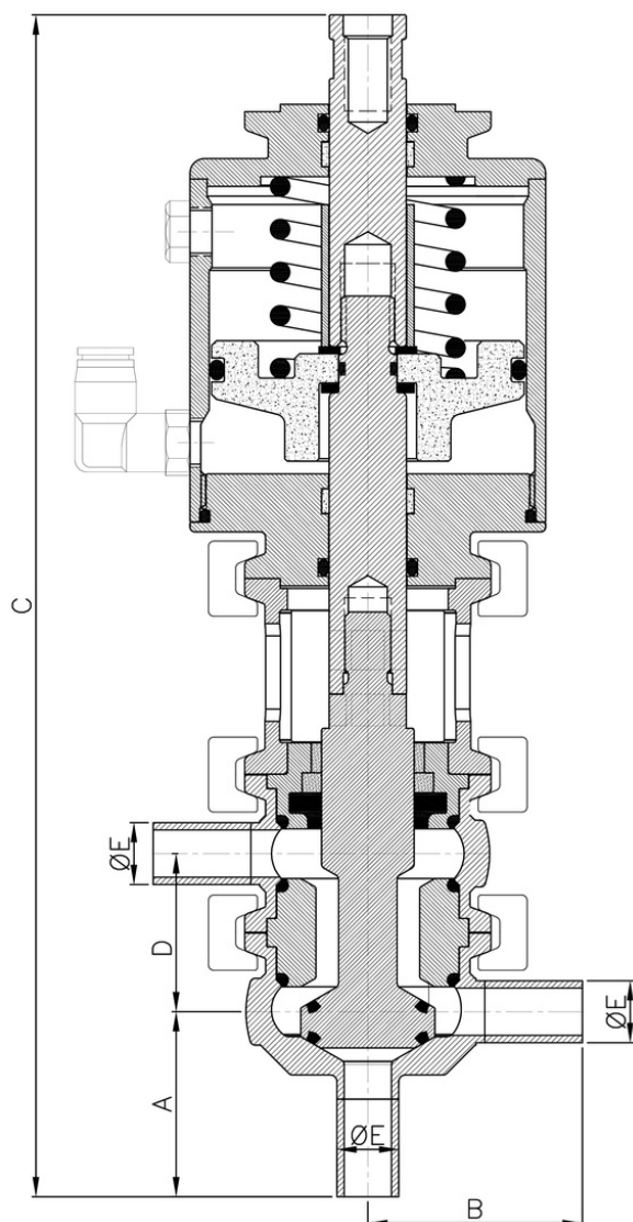
VEH DS CONVERGENTE REBATIBLE Con posibilidad de cabeza de control
