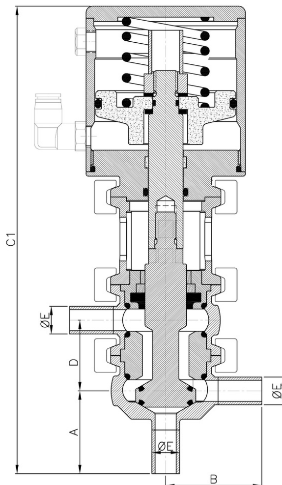
VEH DS CONVERGENTE Sin posibilidad de cabeza de control
