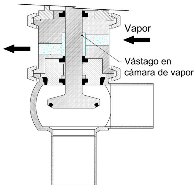
Válvula Abierta (Actuada neumáticamente)
