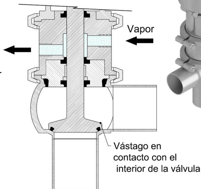
Válvula Cerrada
