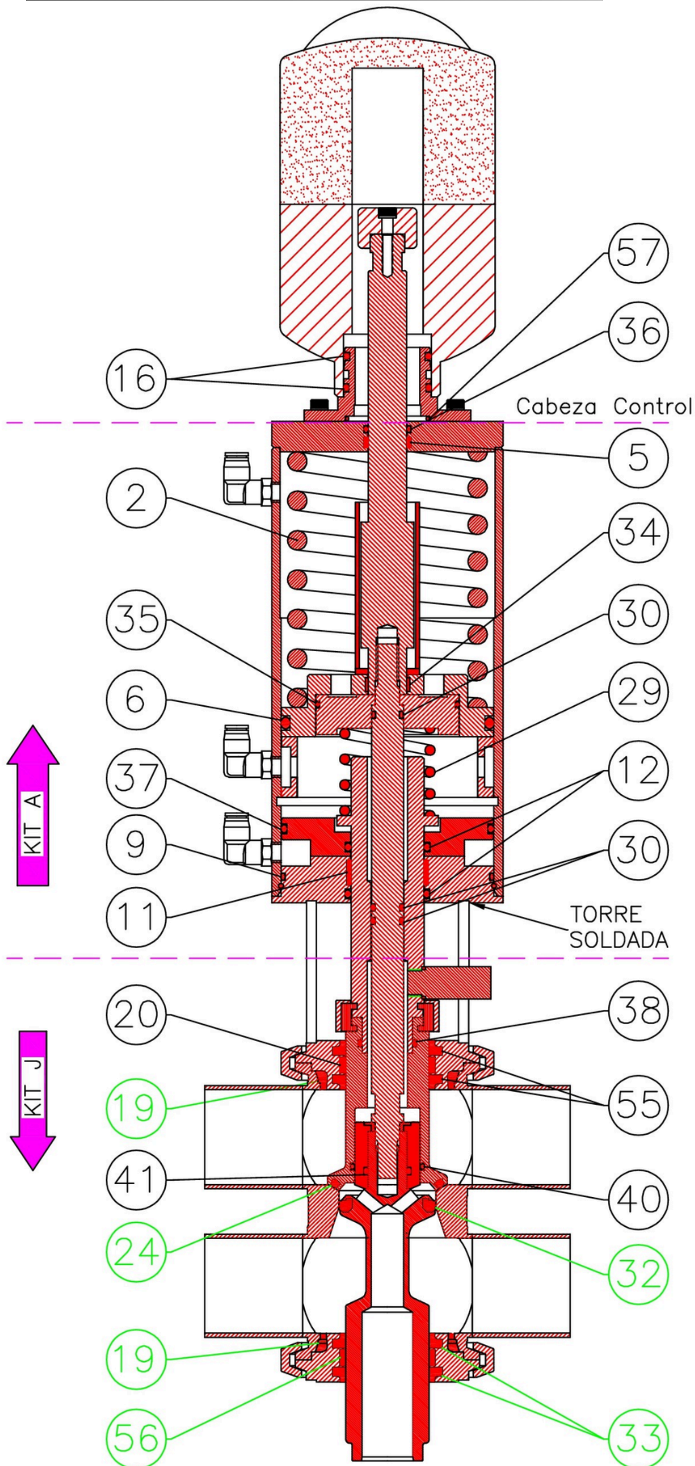
VEH ANT DN MV (torre soldada)
